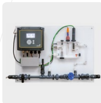
PANELES DE MEDICIÓN Y CONTROL
