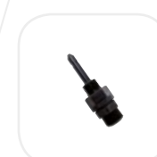
45mm Tubo de 4x6, 6x8, 6x12 y 10x12. Rosca de ½" de PP o PVDF
